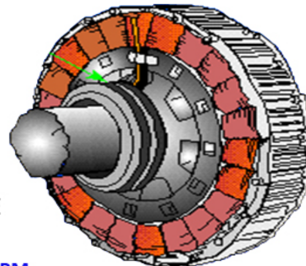
SALIENT-POLE ROTOR
